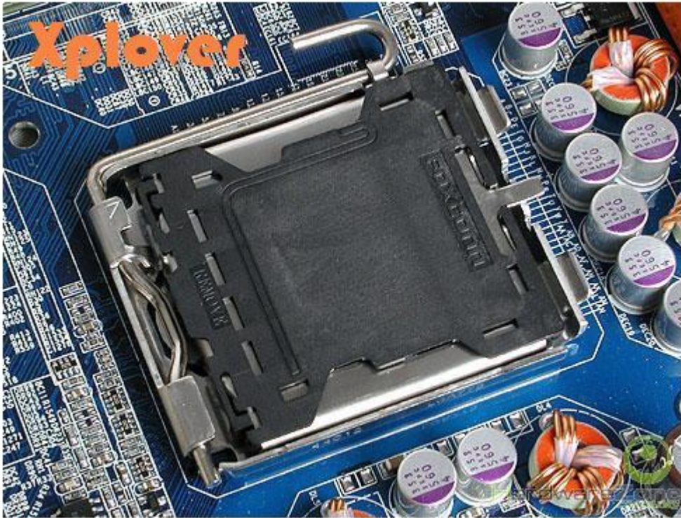
سوکت LGA775 على لوحة الام البنات على السوكت محمية ب غطاء بلاستيك اثناء نقلها
